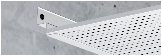
Cornière de rive à joint creux
