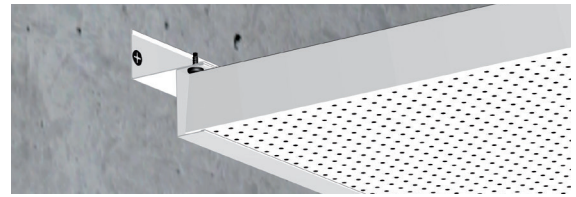
Rive joint creux réglable en deux éléments
